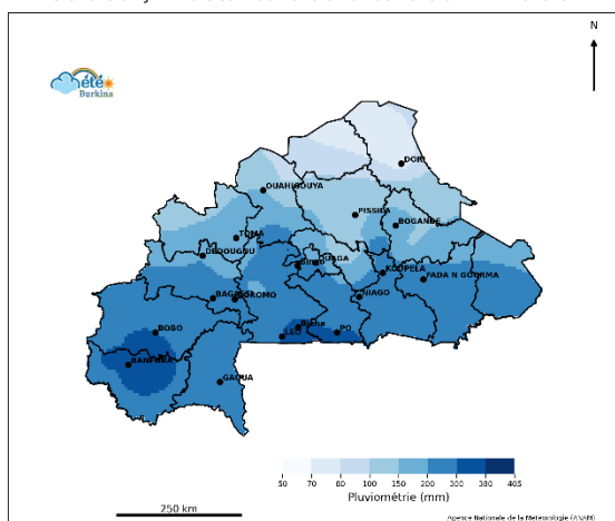
Figure 4 : Cumul saisonnier du 1 avril au 12 juillet 2026
