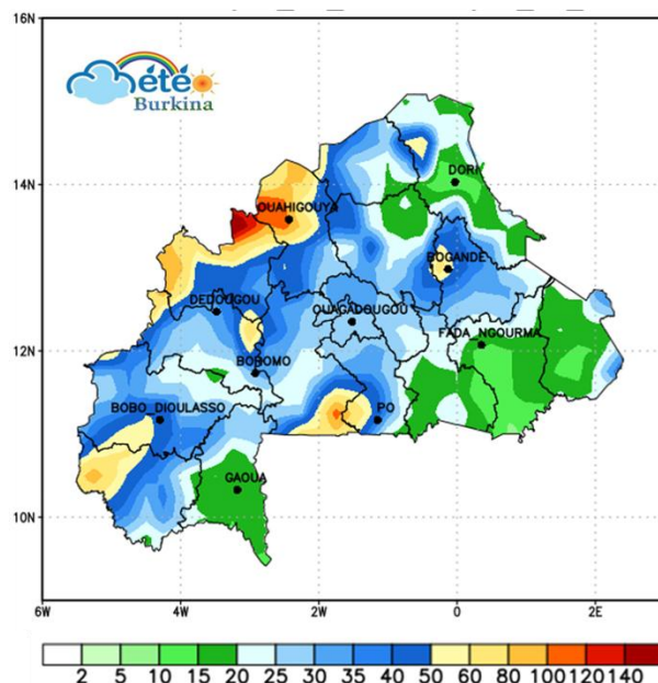
Figure 6 : Cumuls pluviométriques du 13 au 19 juillet 2026. Source NOAA GFS
