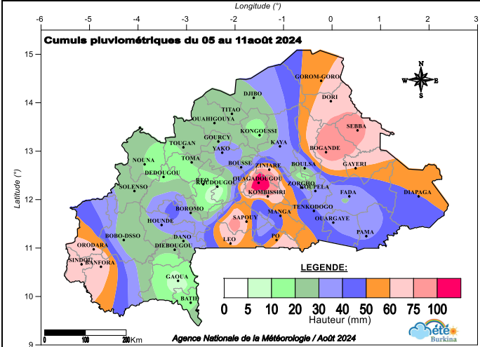
Figure 2 : cumuls pluviométriques du 05 au 11 août 2024
