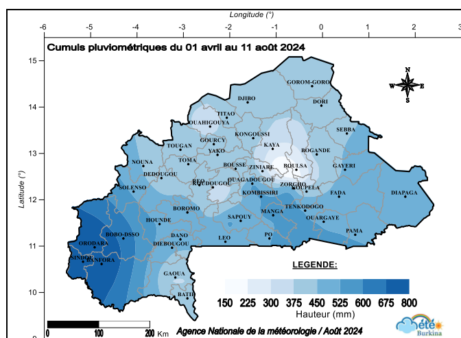
Figure 4 : cumuls pluviométriques du 1 er avril au 11 août 2024
