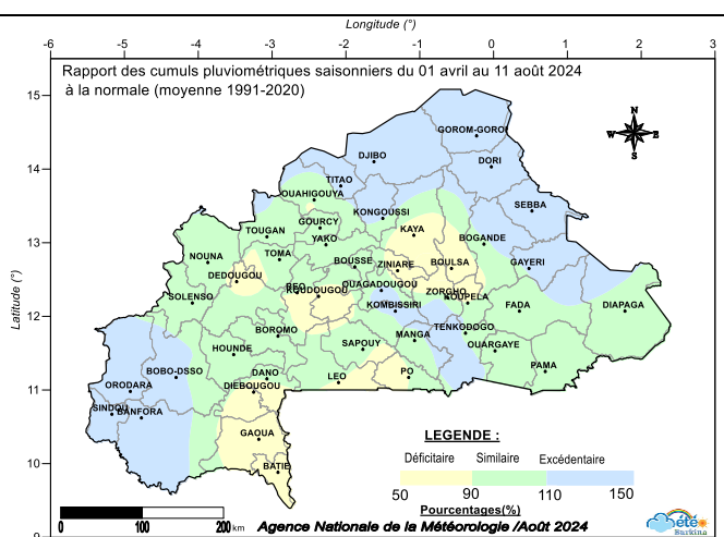
Figure 5 : cumuls pluviométriques du 1 er avril au 11 août 2024 comparés à la normale 1991-2020
