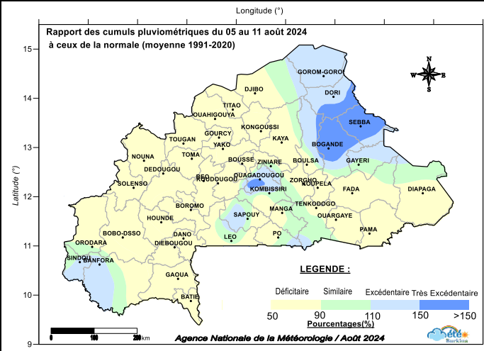
Figure 3 : cumuls pluviométriques du 05 au 11 août 2024 comparés à la normale 1991-2020
