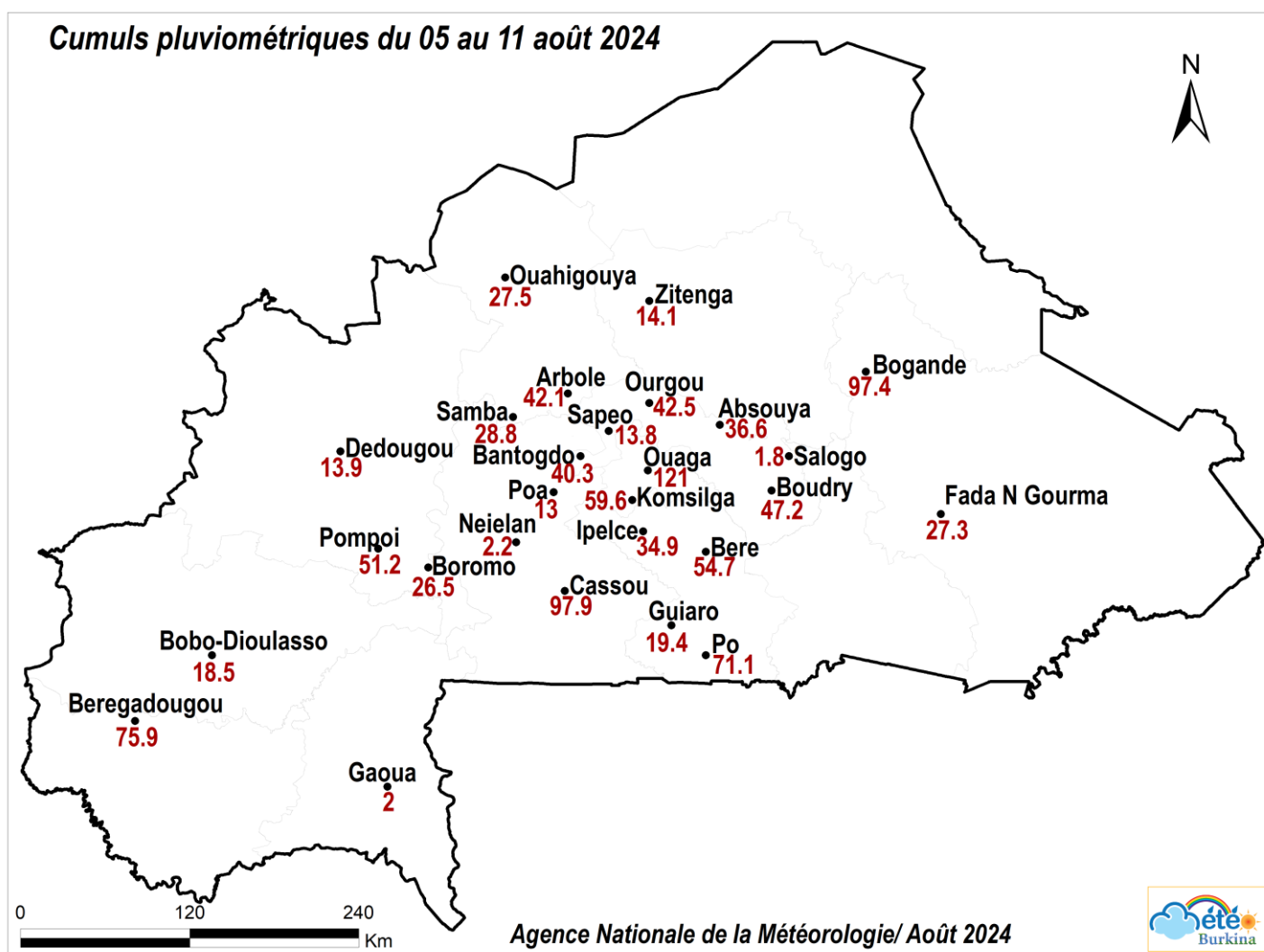
Figure 1 : cumuls pluviométriques du 05 au 11 août 2024
