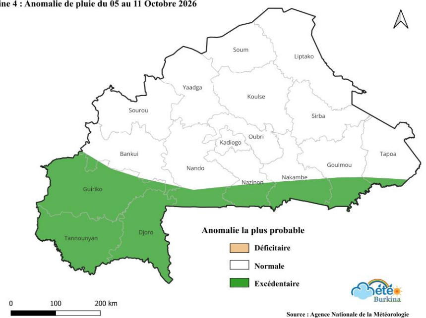
Semaine 4 : Anomalie de pluie du 05 au 11 Octobre 2026
