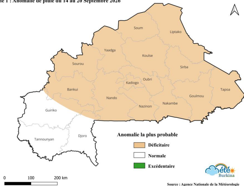
Semaine 1 : Anomalie de pluie du 14 au 20 Septembre 2026
