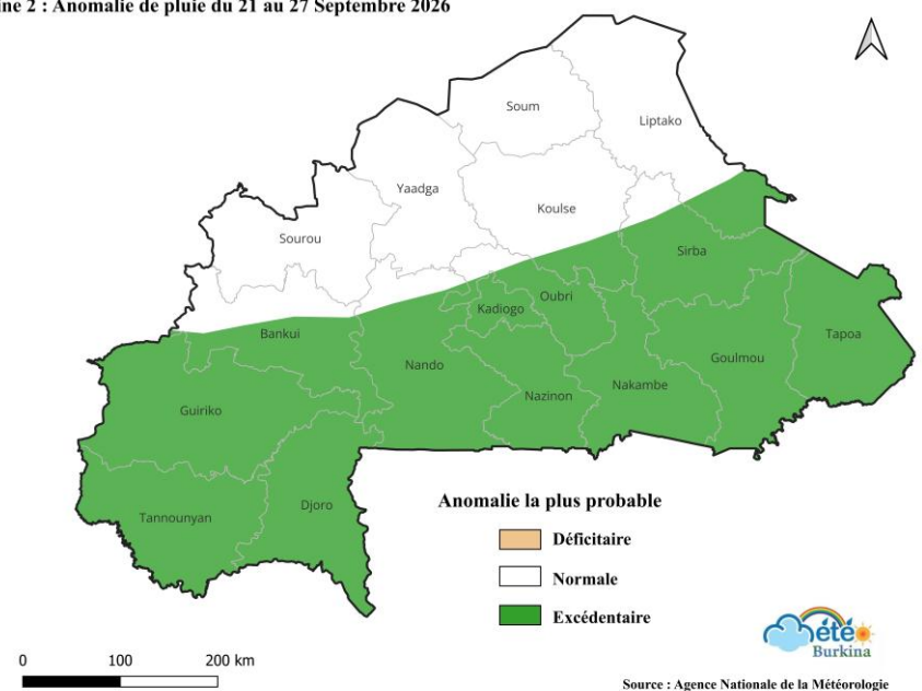
Semaine 2 : Anomalie de pluie du 21 au 27 Septembre 2026
