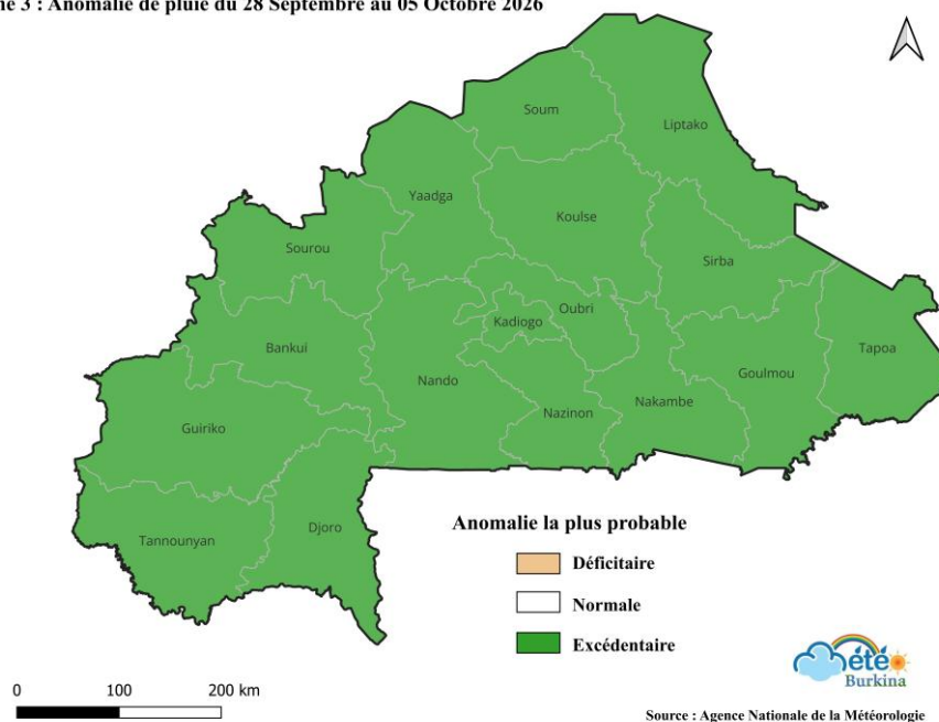
Semaine 3 : Anomalie de pluie du 28 Septembre au 05 Octobre 2026
